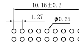
P.C.B LAYOUT
